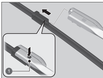
1 Príchytka
