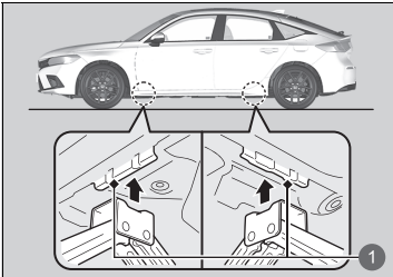
1 Zdvíhacie body
